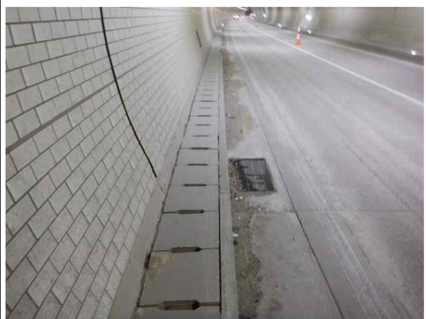
공동구 및 배수구 전경
